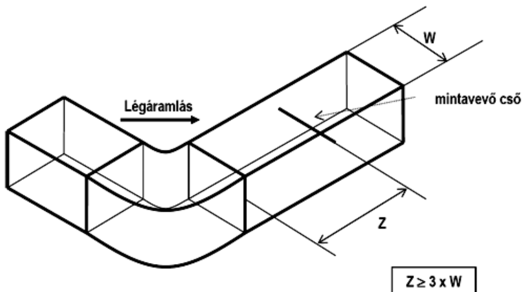
Légcsatorna érzékelő elhelyezése légcsatorna görbületnél
