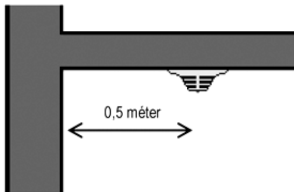
Pontszerű érzékelő elhelyezése gerendák (kötényfalak) mellett
