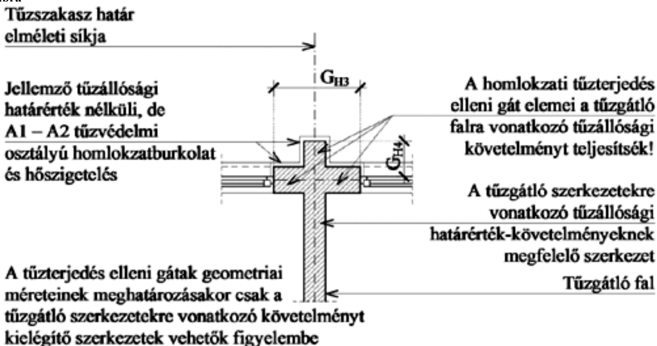
Vízszintes homlokzati tűzterjedés elleni gát metszete
