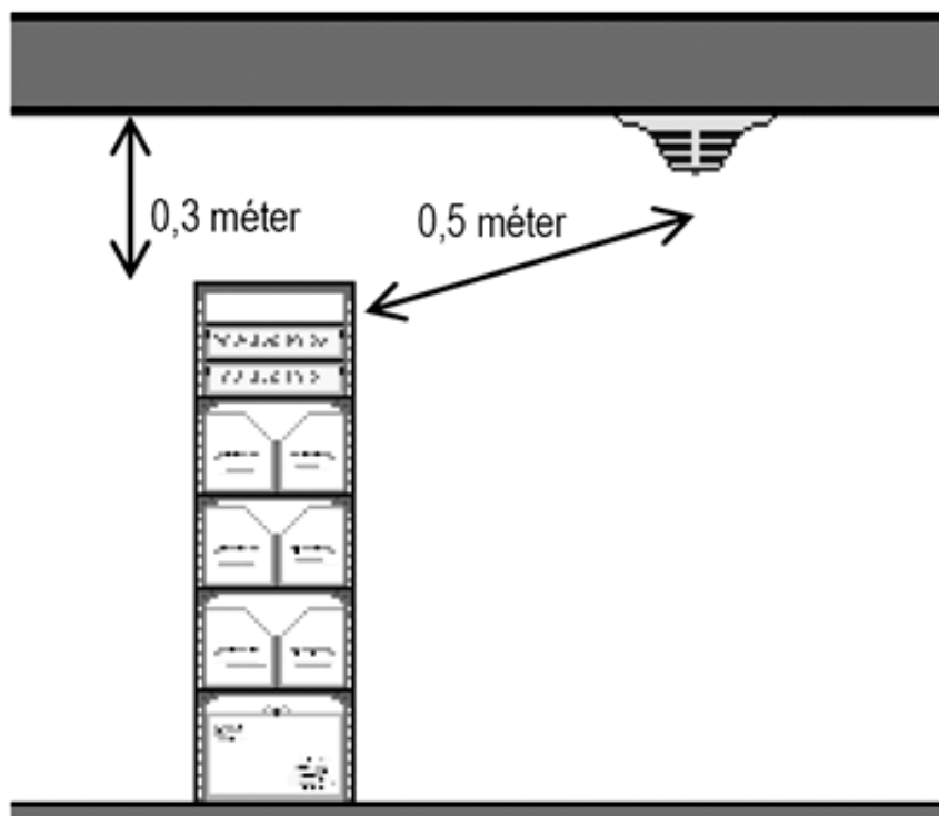
Pontszerű érzékelő elhelyezése épületgépészeti elem mellett
