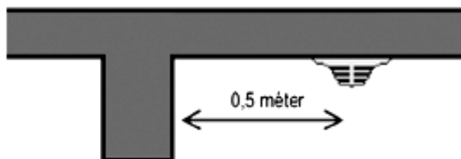
Pontszerű érzékelő elhelyezése polcos tárolás esetében
